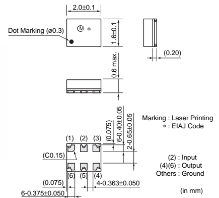
SAFEH2G14FA0F00
